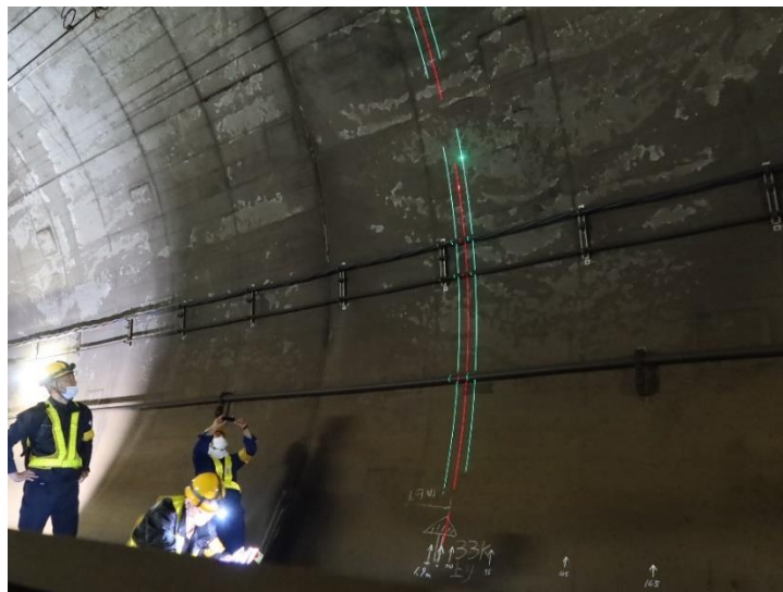
図1 内空断面の計測状況
