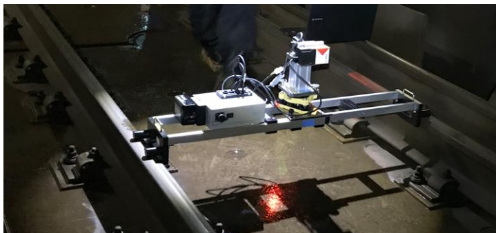
図2 断面測定器
